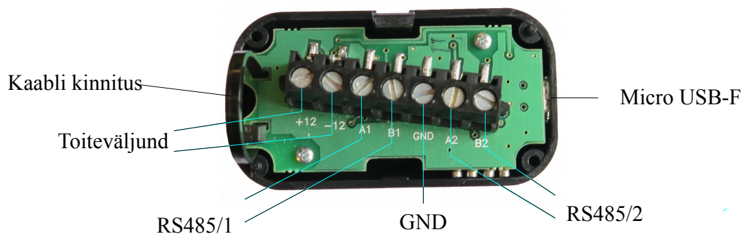
Joon 1. Vaade avatud kateaga. Kontaktid ja ühendused.
