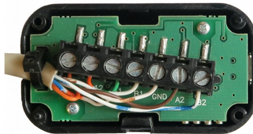
Joon 2. Vaade avatud kateaga. Kaabli kinnitus.
