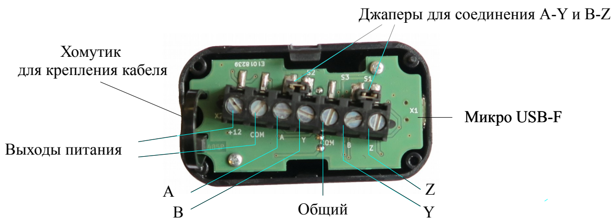
Рис. 1. Вид со снятой крышкой. Назначение соединителей
