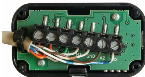
Рис. 2. Вид со снятой крышкой. Крепление кабеля
