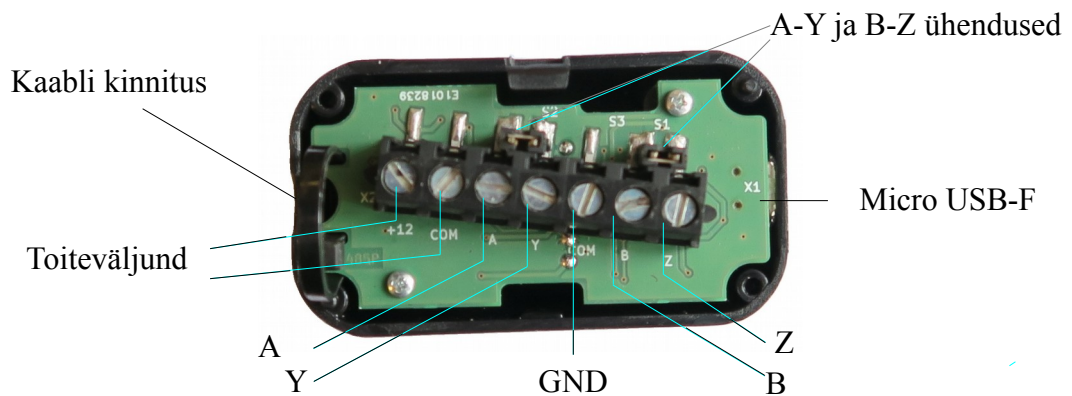
Joon 1. Vaade avatud kateega. Kontaktid ja ühendused.
