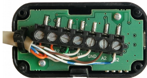
Joon 2. Vaade avatud kateega. Kaabli kinnitus.
